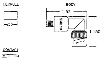
DIMENSIONS \Delta
