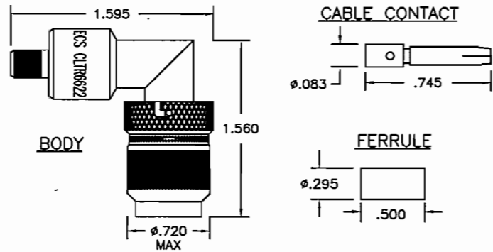
DIMENSIONS 4
